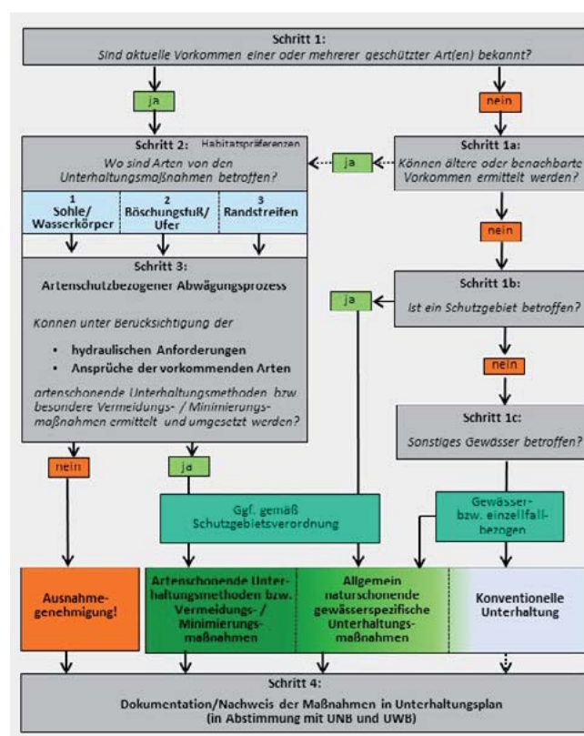
Prüf- und Ablaufschema nach NLWKN (2017)
